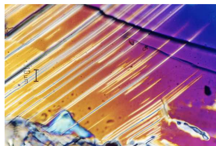
Macles de déformation dans une stishovite (quartz de très haute pression)
