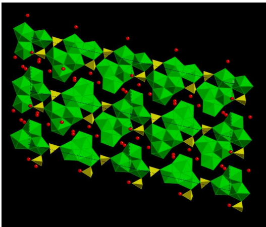
Structure cristalline d'un nouveau minéral d'uranium des Marécottes, VS
