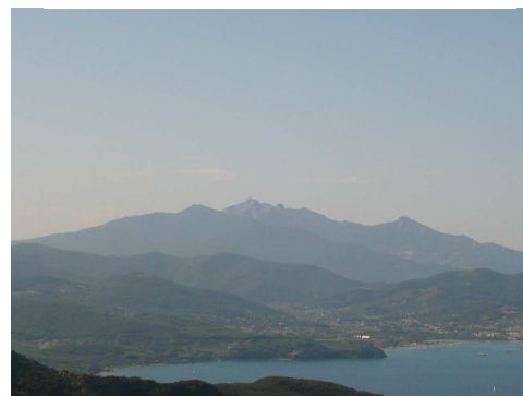
Intrusion du Mte. Capanne
